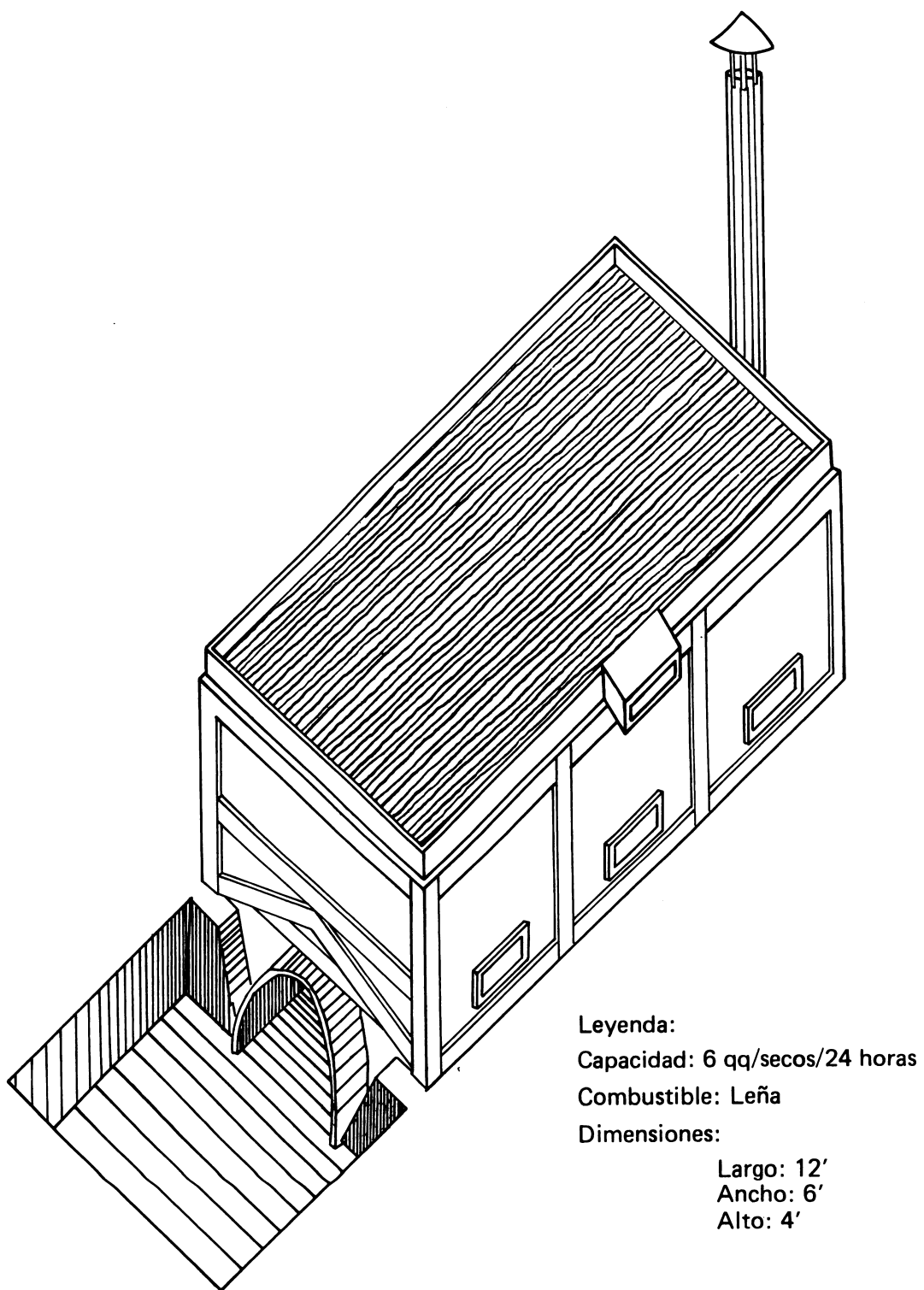
Fig. 4. Secadora de Cacao Modelo APC-03.
