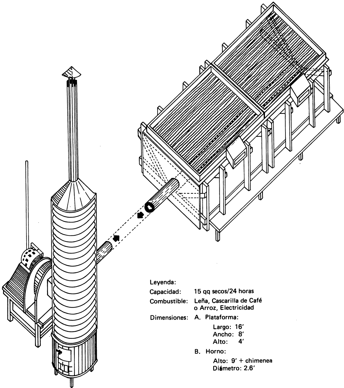
Fig. 5. Secadora de Cacao Modelo APC-04E.
