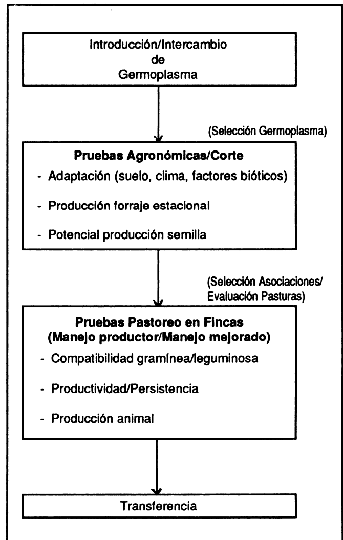
Figura 4. Modelo Alternativo C de evaluación de Germoplasma/Pasturas.
