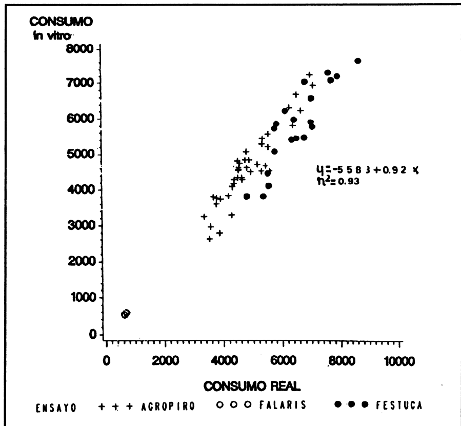
Figura 17. Relación entre el consumo real y el calculado por digestibilidad in vitro . Rosso et al. (1990)
