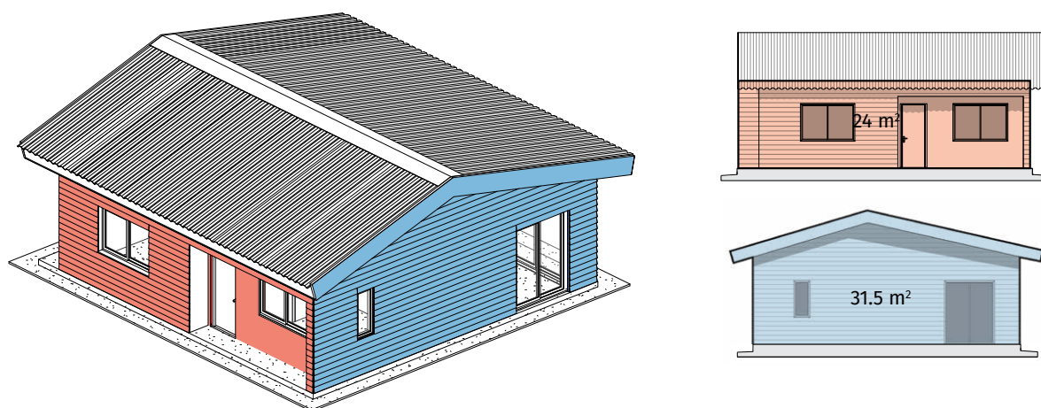
FIGURA 3.7. Cuantificación de la superficie expuesta al viento de la vivienda según las 2 direcciones principales
