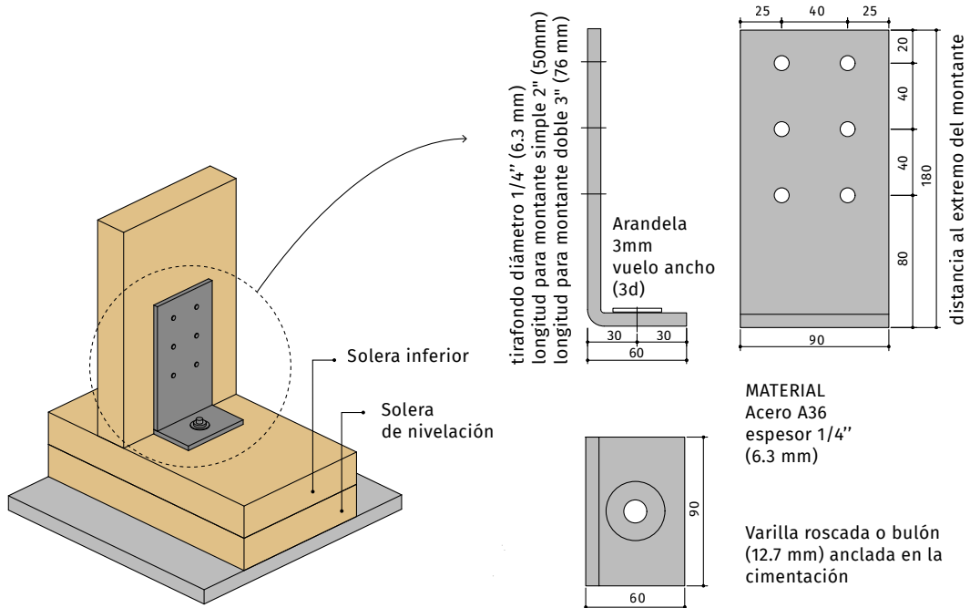
FIGURA 4.23 Anclaje de montantes que no están ubicados en los extremos de muros de corte
