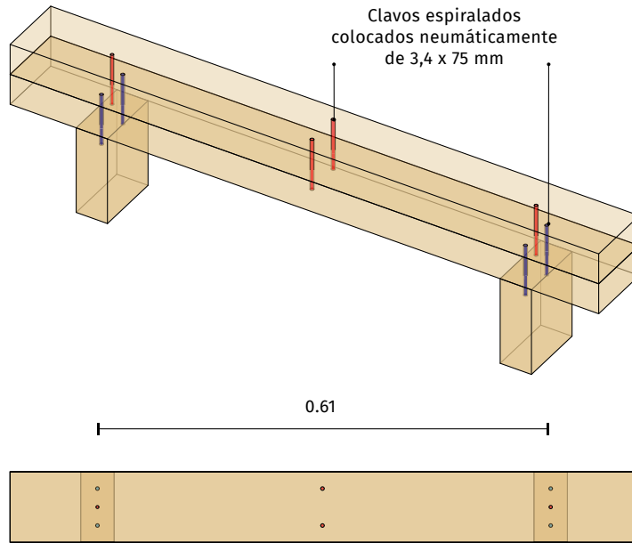
FIGURA 3.34 B. Unión entre la solera superior y los montantes y entre ambas soleras
