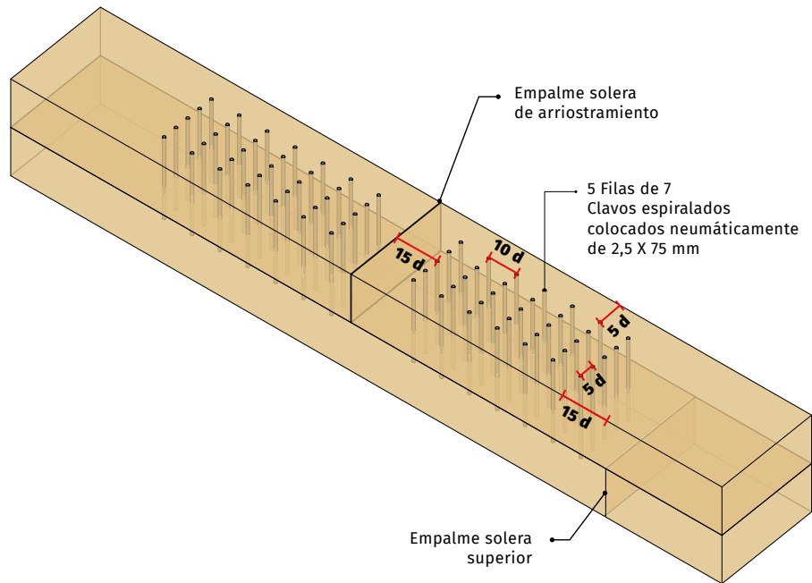
FIGURA 4.32. Empalme de una pieza de borde
