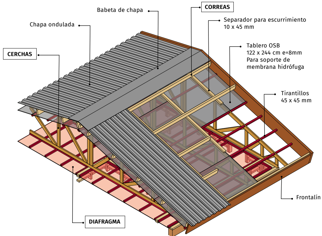
FIGURA 3.9. Disposición general de los componentes de la cubierta
