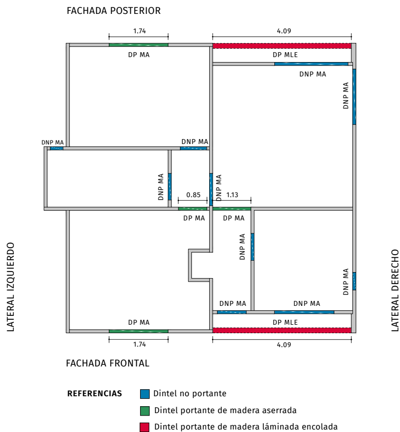
FIGURA 3.16. Identificación de dinteles
