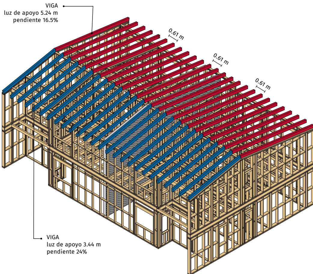
FIGURA 4.4 Esquema general de la estructura de la cubierta
