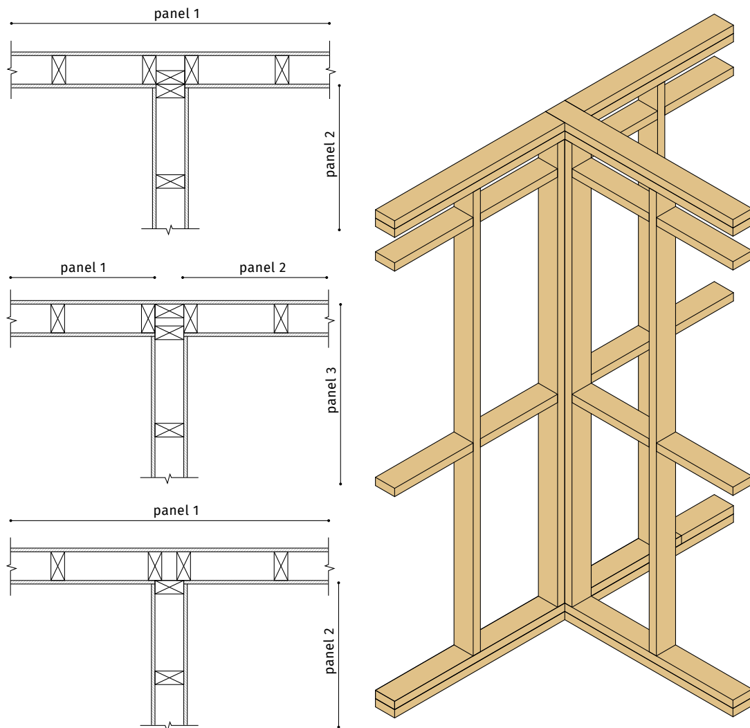
FIGURA 4.35 A1 Posibles soluciones de encuentros entre muros
