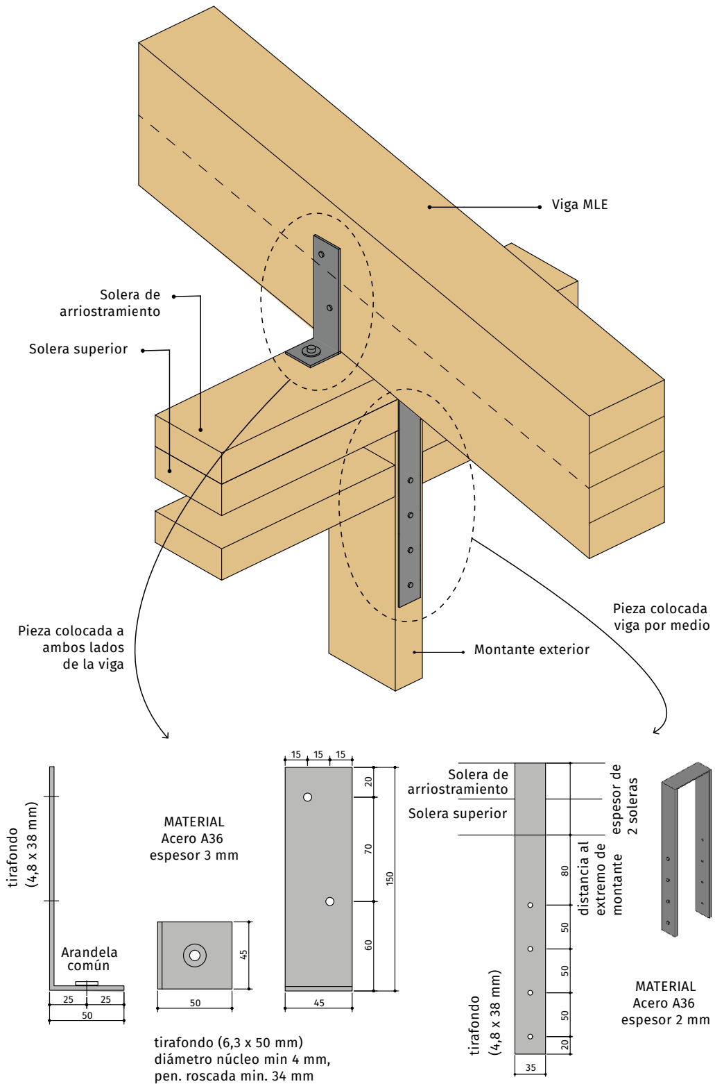
FIGURA 4.18 Detalle de la unión viga de techo - solera y solera - montante sobre los muros de ambas fachadas
