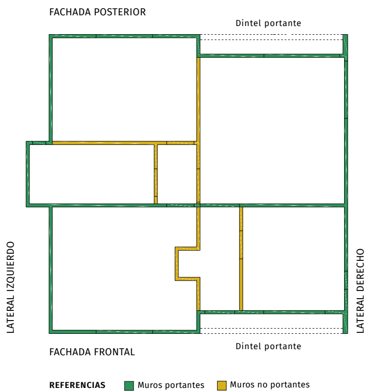
FIGURA 3.6. Identificación de la función estructural de los muros
