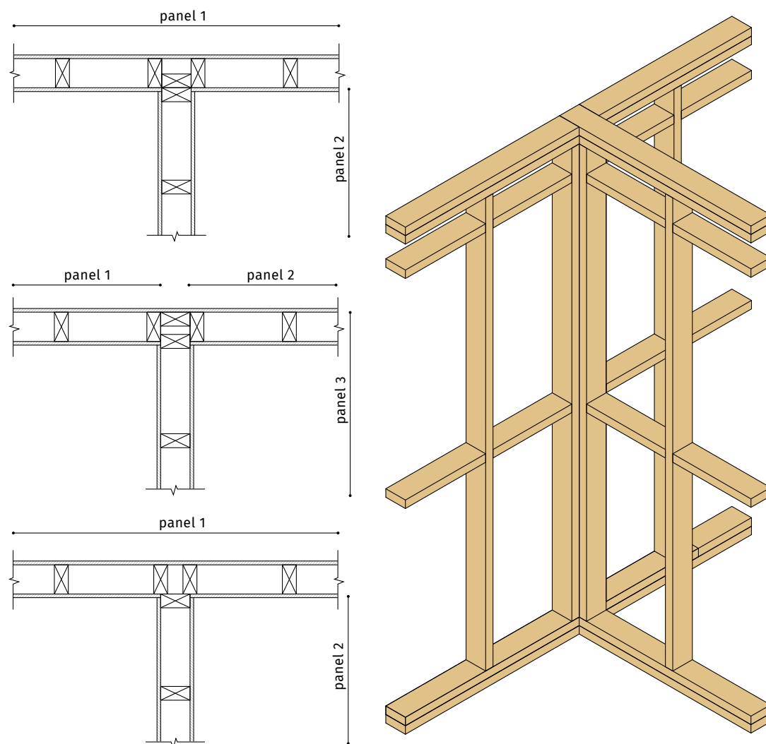
FIGURA 3.34 A2. Posibles soluciones de encuentro entre muros
