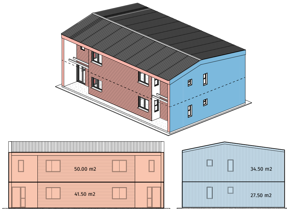
FIGURA 4.9 Cuantificación de la superficie expuesta al viento de la vivienda según las dos direcciones principales
