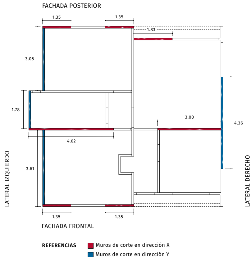
FIGURA 3.8. Longitud de los muros de corte
