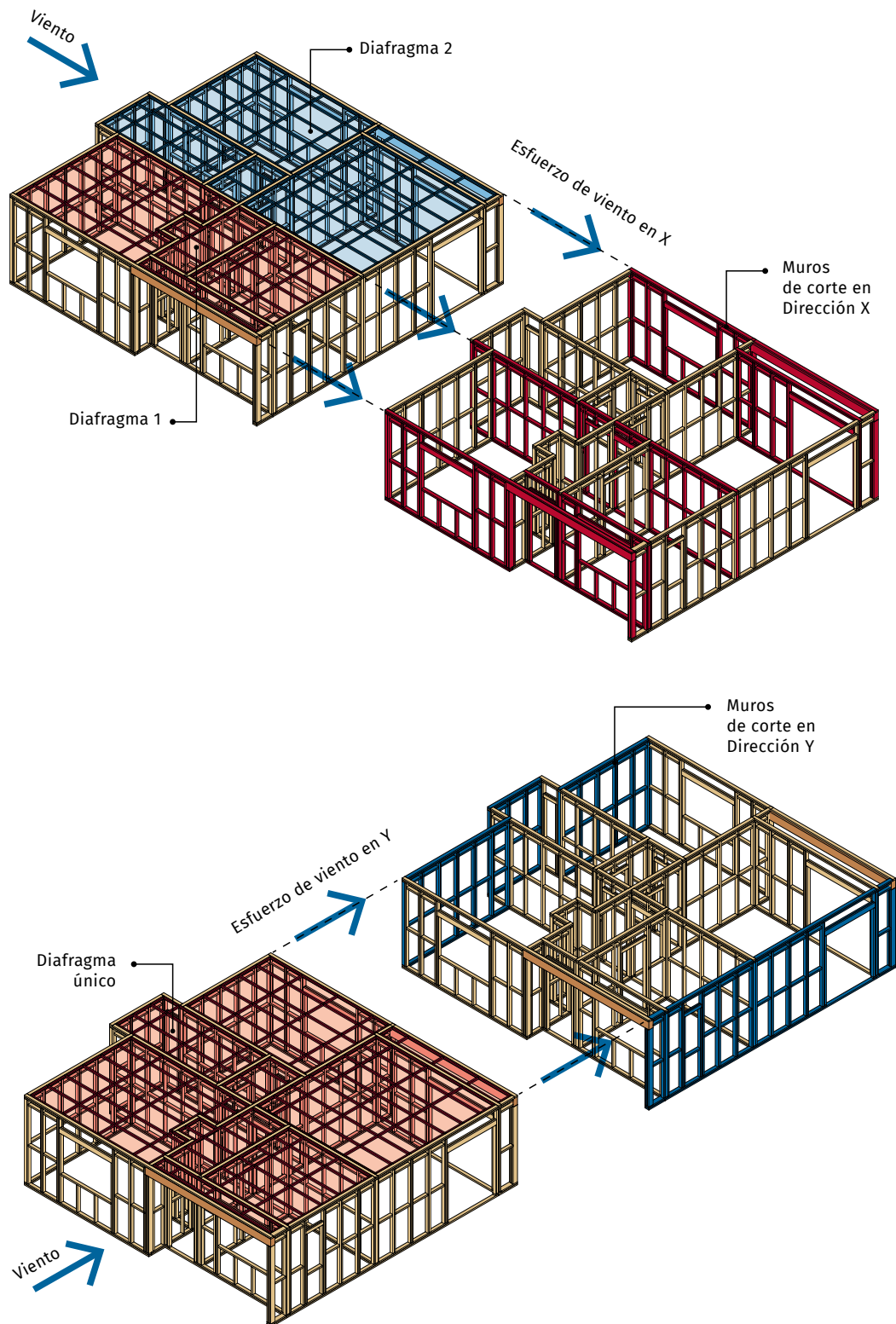
FIGURA 3.5. Características generales del diafragma horizontal
