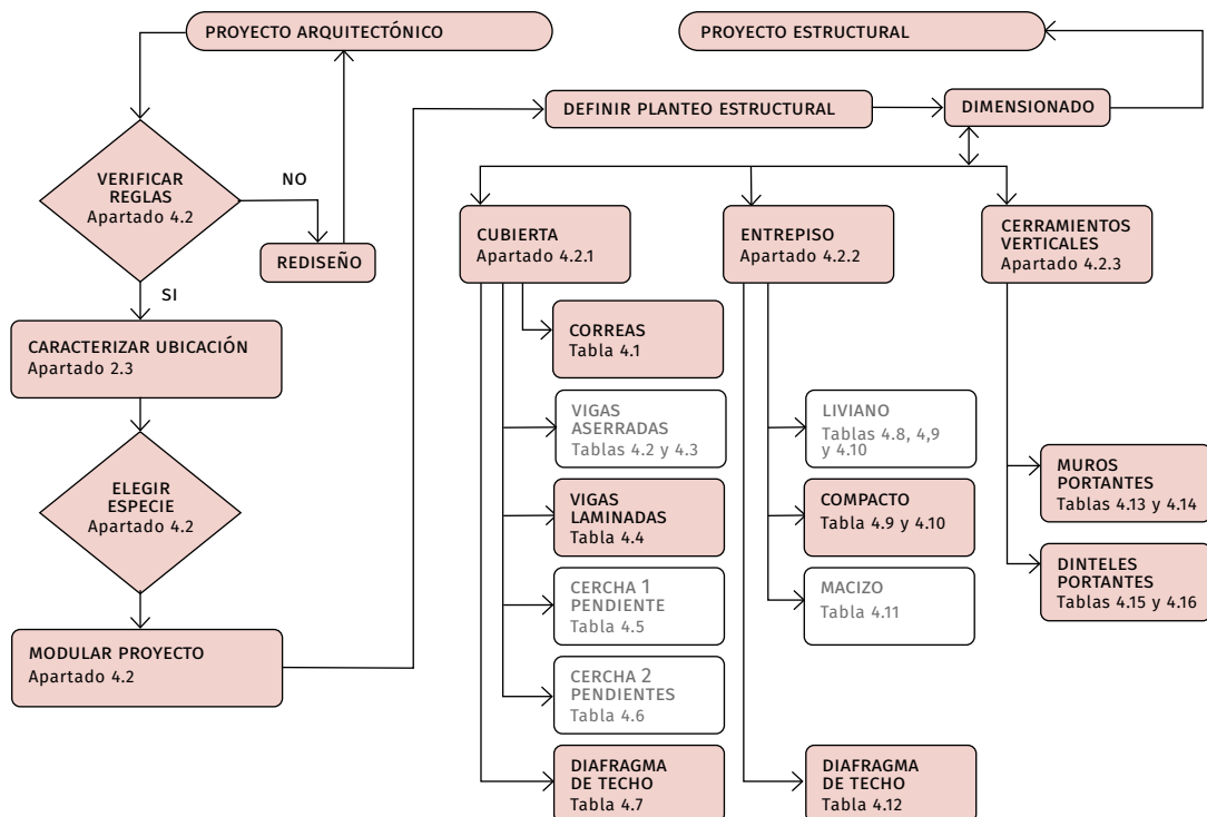
FIGURA 4.1 Diagrama de flujo del procedimiento adoptado para resolución del modelo
