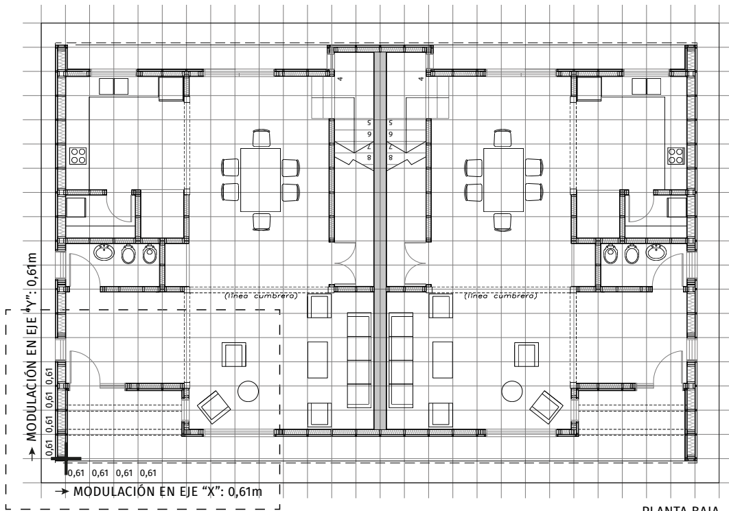
DETALLE: Distribución de montantes de acuerdo a la modulación
