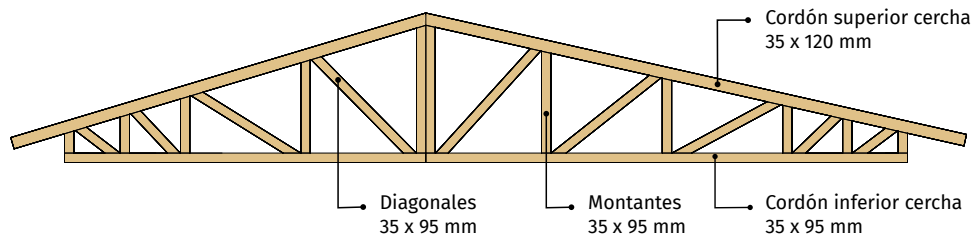
FIGURA 3.11. Características generales de las cerchas adoptadas
