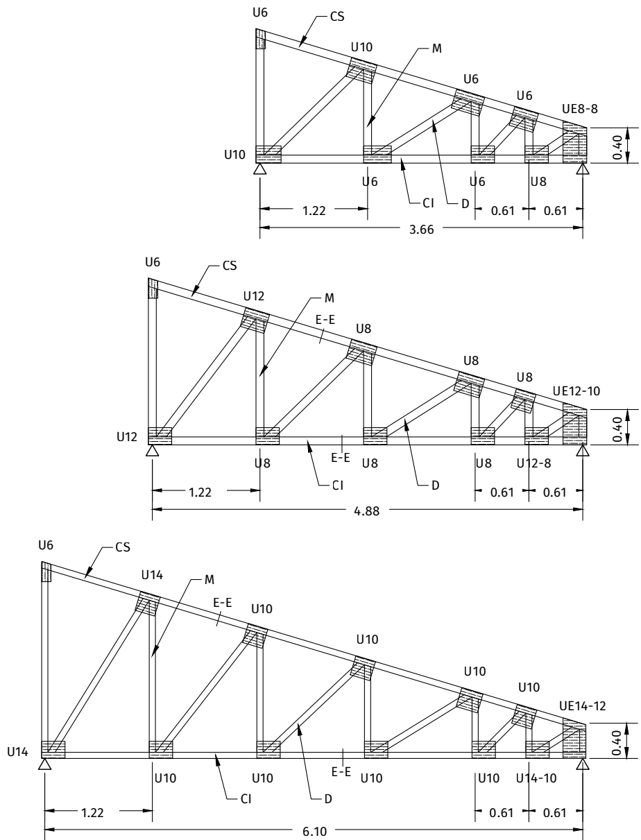
FIGURA 4.25 Descripción general de las cerchas con una pendiente
