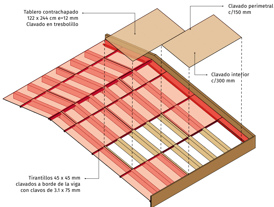
FIGURA 4.13 Detalle de la conformación del diafragma de la cubierta
