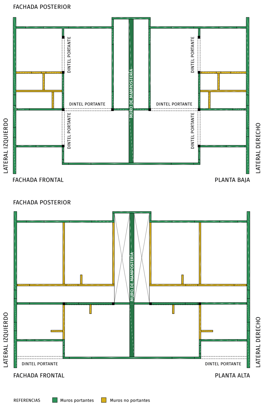
FIGURA 4.8 Identificación de la función estructural de los muros
