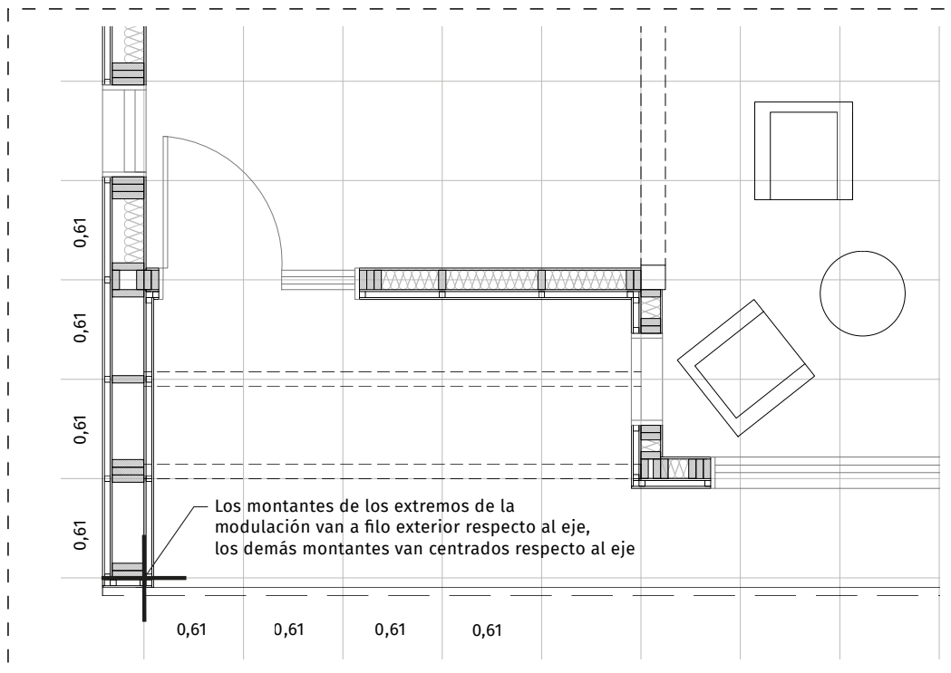
FIGURA 4.3 Modulación del entramado estructural
