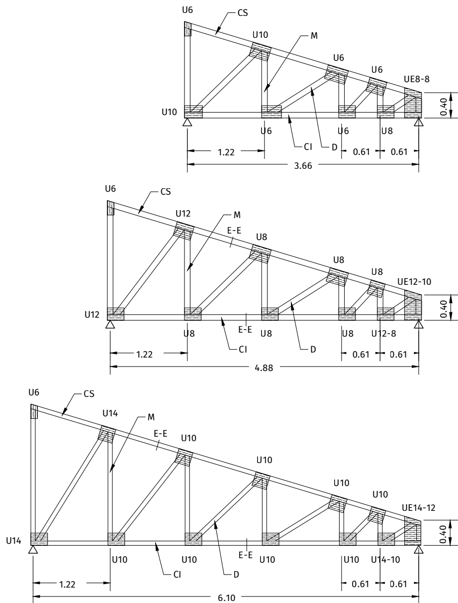
FIGURA 3.24. Descripción general de las cerchas con una pendiente
