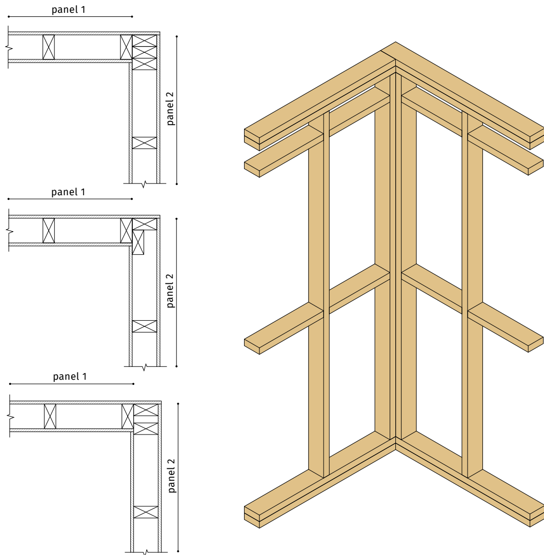
FIGURA 3.34 A1. Posibles soluciones de encuentro entre muros
