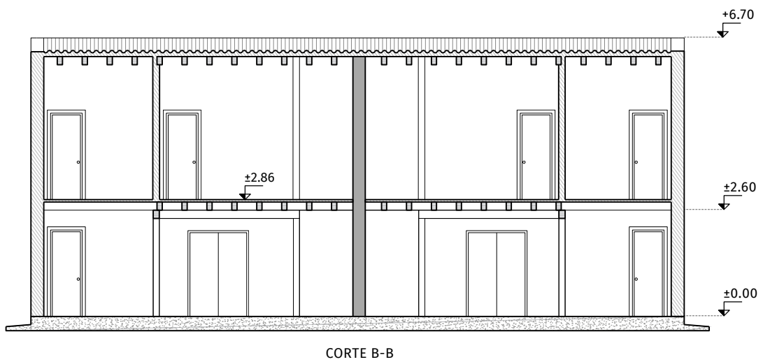
FIGURA 4.2 E Cortes
