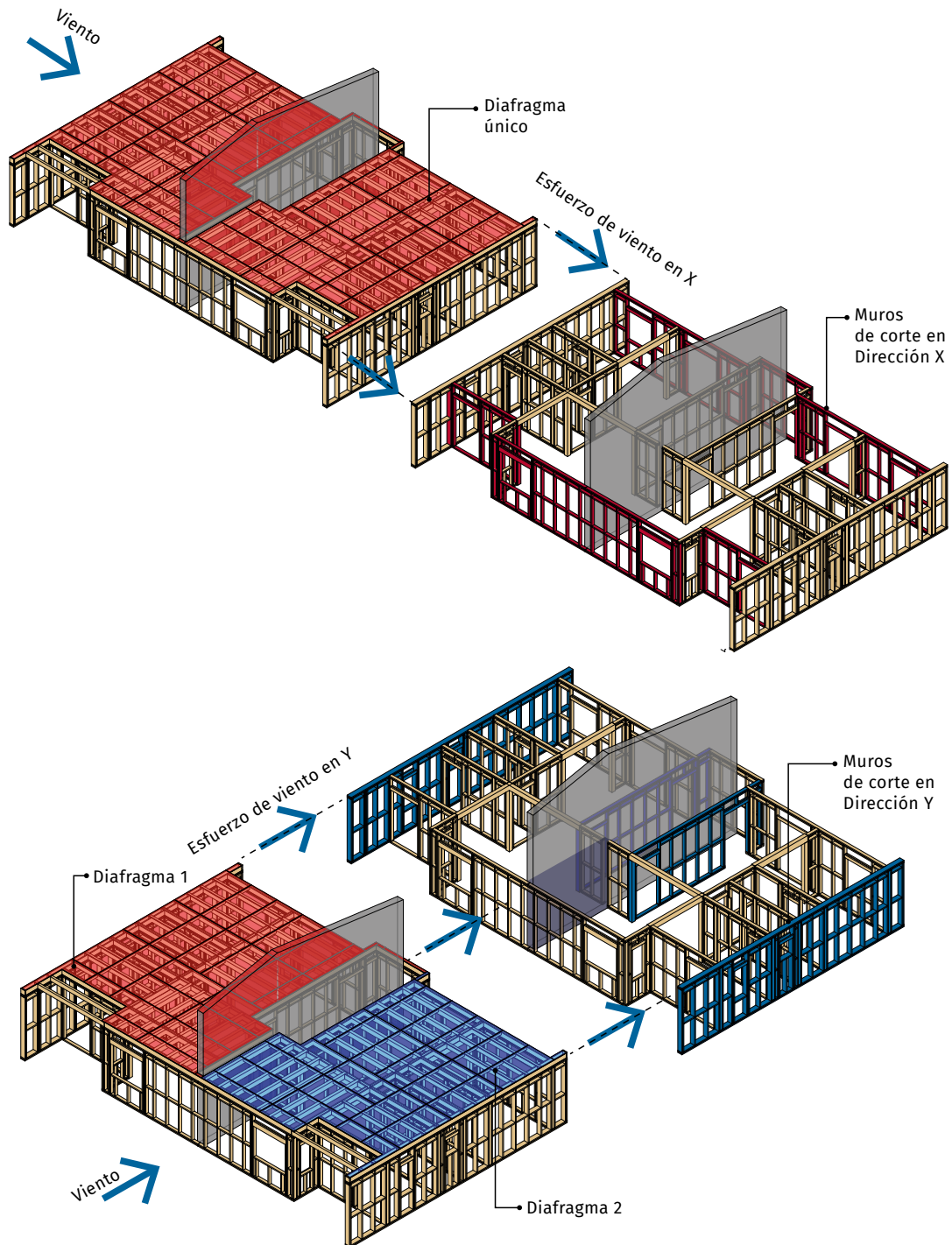
FIGURA 4.7 Características generales del diafragma de entrepiso
