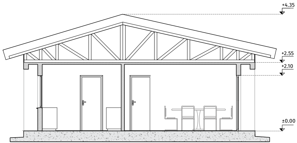
CORTE A-A
