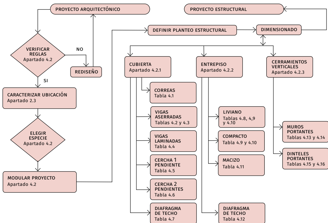
FIGURA 4.24 Diagrama de flujo del procedimiento general para resolución de la estructura
