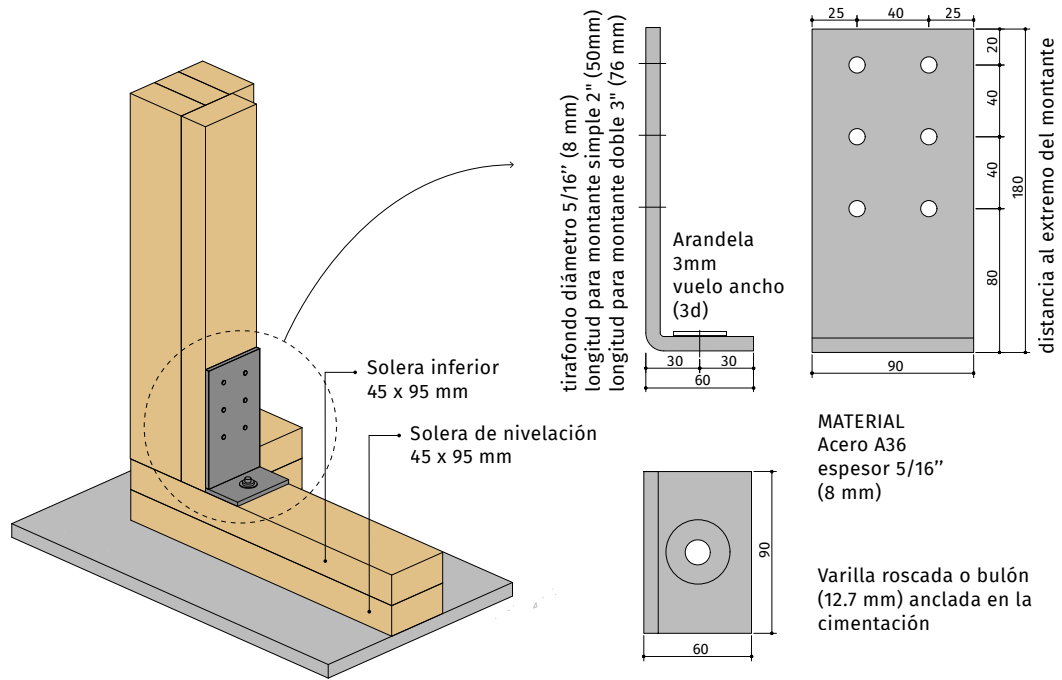
FIGURA 3.21. Anclaje de montantes extremos en los muros de corte
