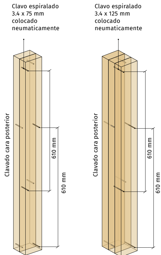
FIGURA 3.32. Unión de montantes constituidos por más de una pieza
