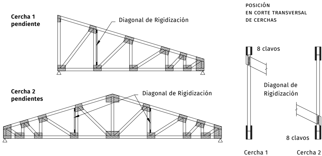
FIGURA 4.29 Rigidización transversal de las cerchas
