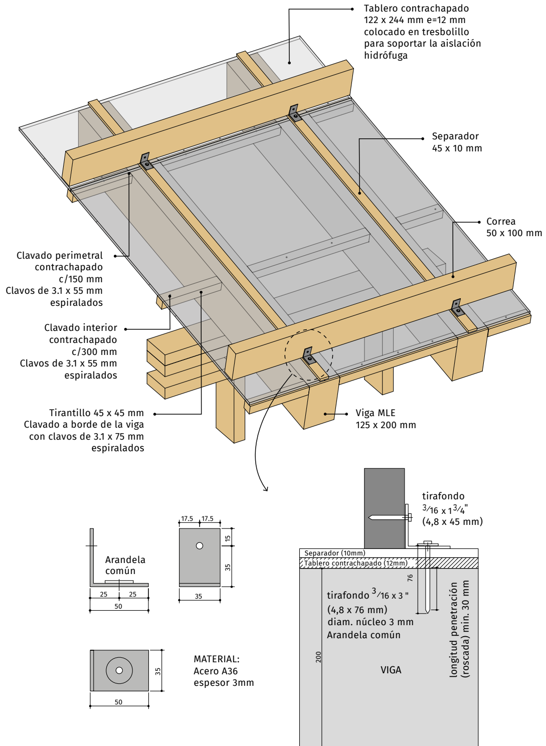
FIGURA 4.12 Detalle de la colocación de las correas y su unión a las vigas de cubierta
