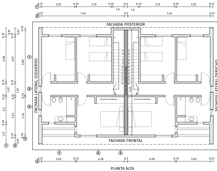
FIGURA 4.2 C Planta Alta
