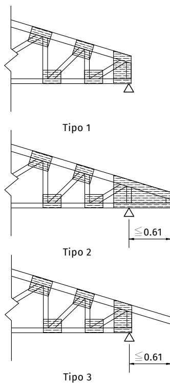
FIGURA 4.27 Tipologías de extremos
