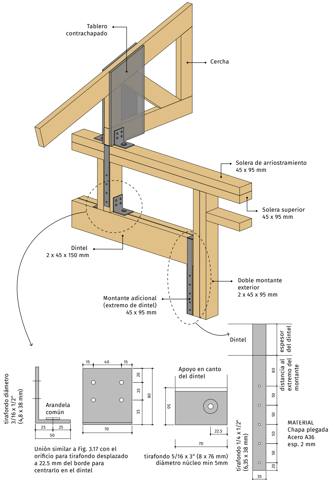
FIGURA 3.18. Detalle de apoyo de cercha sobre dintel
