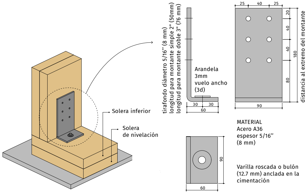
FIGURA 4.22 Anclaje de montantes extremos en los muros de corte
