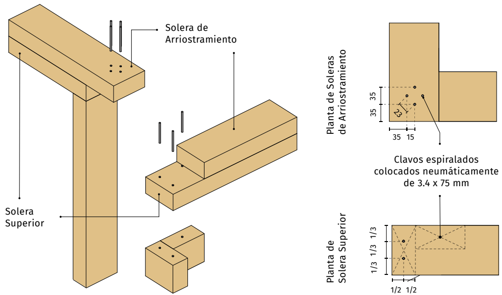
FIGURA 3.34 C. Clavadura de solera a montantes y entre soleras en esquina
