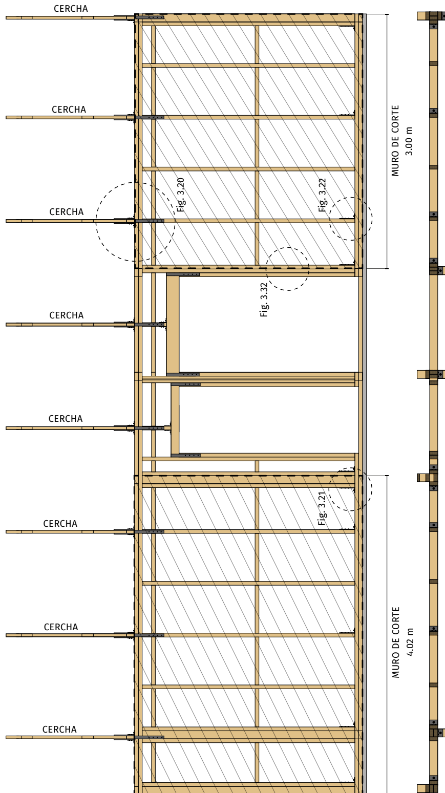
FIGURA 3.15. Conformación del muro portante interior donde apoya la cubierta
