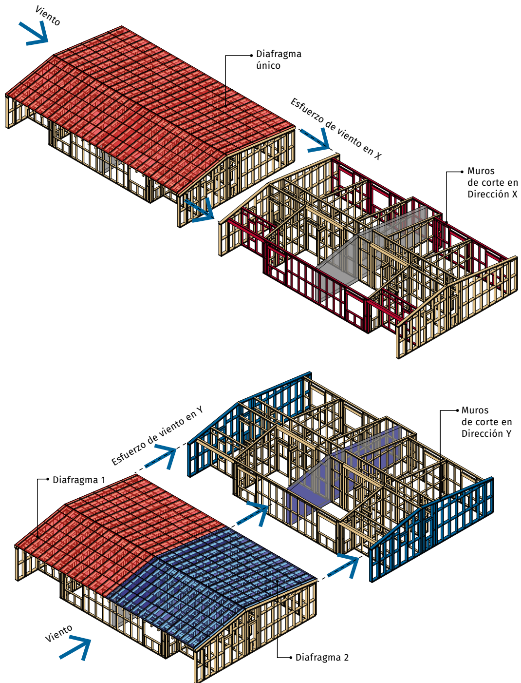
FIGURA 4.5 Características generales del diafragma de cubierta
