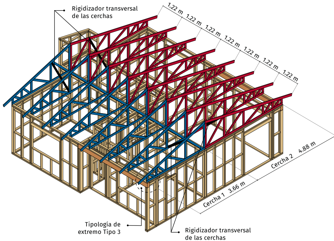
FIGURA 3.4. Estructura de la estructura de la cubierta
