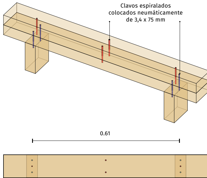
FIGURA 4.35 B. Unión entre la solera superior y los montantes y entre ambas soleras
