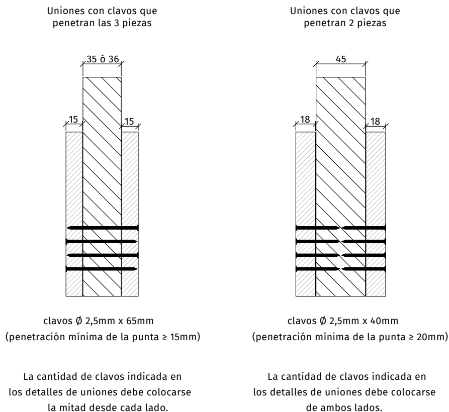
FIGURA 3.30. Características de las conexiones
