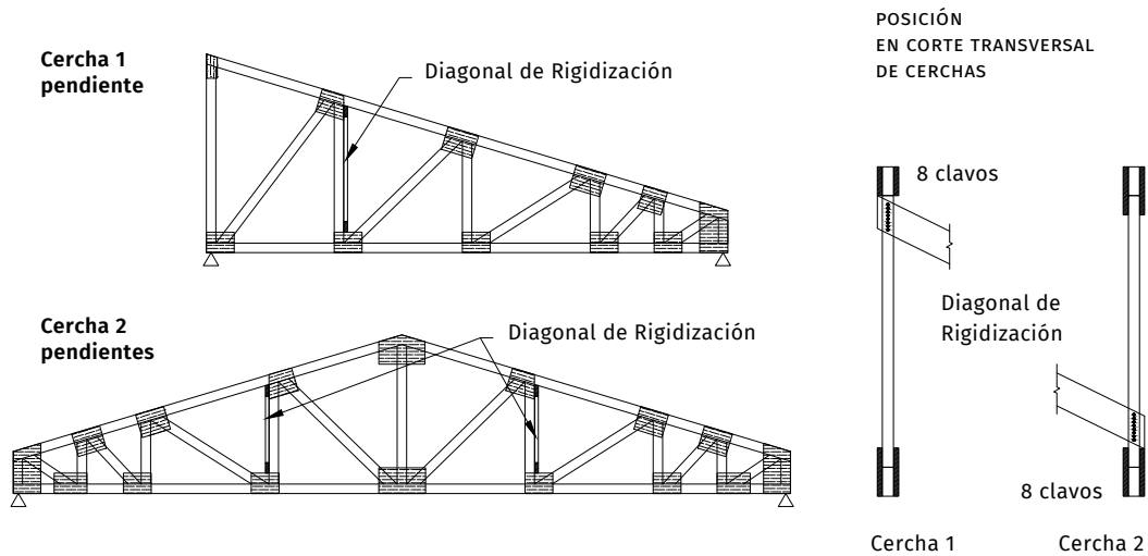
FIGURA 3.28. Rigidización transversal de las cerchas
