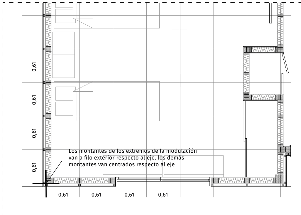
FIGURA 3.3. B. Modulación de entramado estructural
