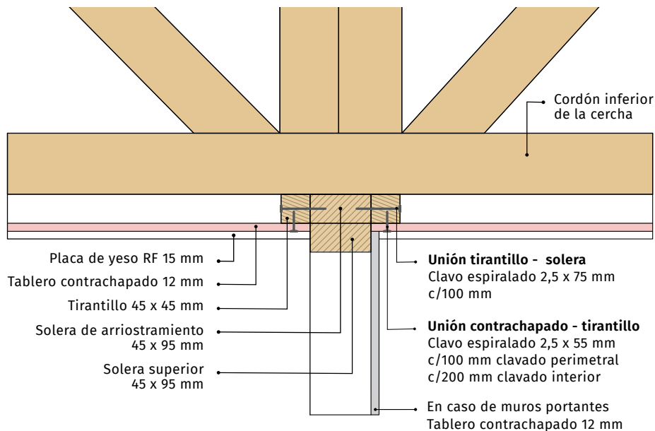
FIGURA 3.13. Continuidad del diafragma a través de muros interiores
