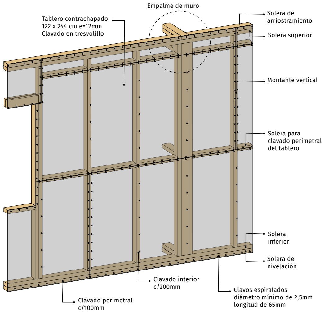
FIGURA 3.33. Clavado de los tableros a las soleras y montantes
