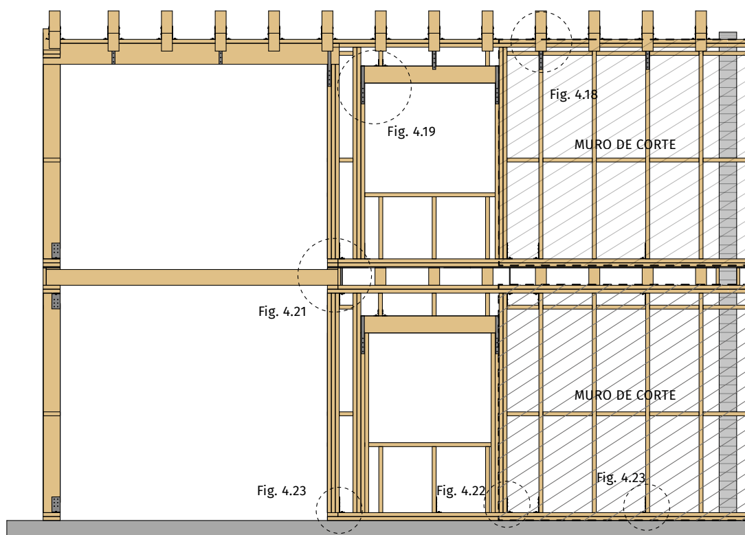
FIGURA 4.15 Conformación del muro de la fachada frontal
