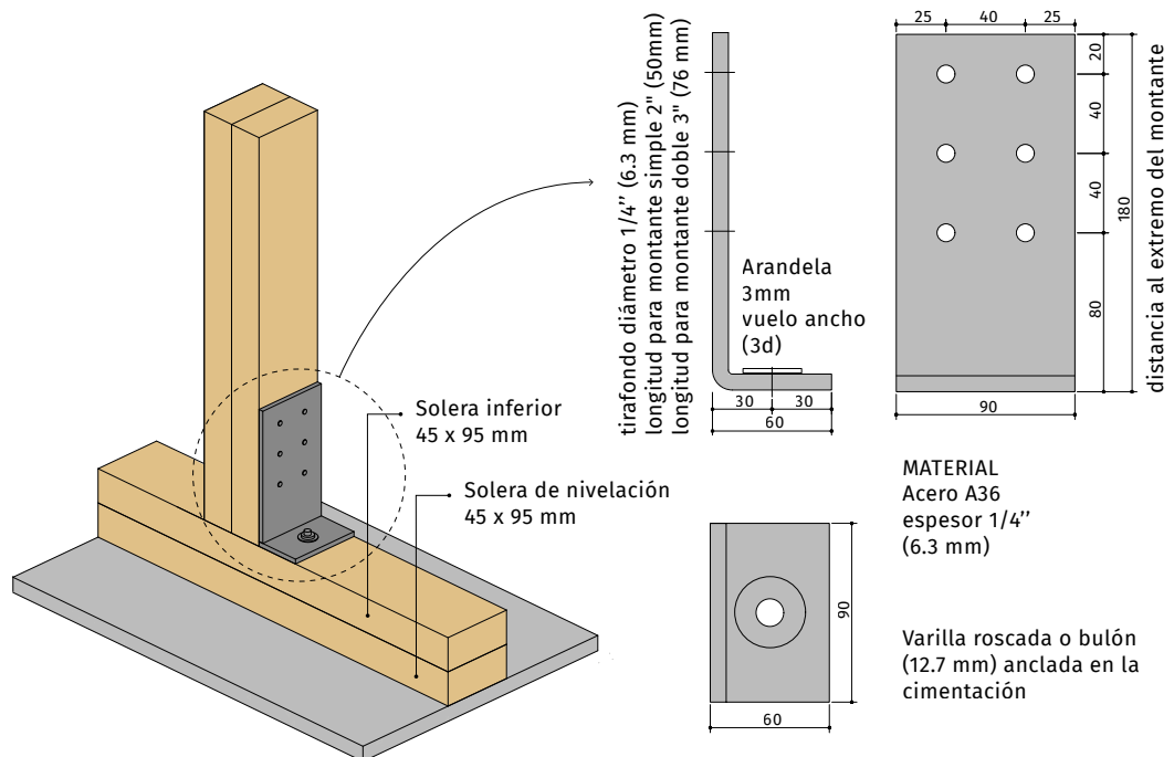
FIGURA 3.22. Anclaje de montantes que no están ubicados en los extremos de los muros de corte
