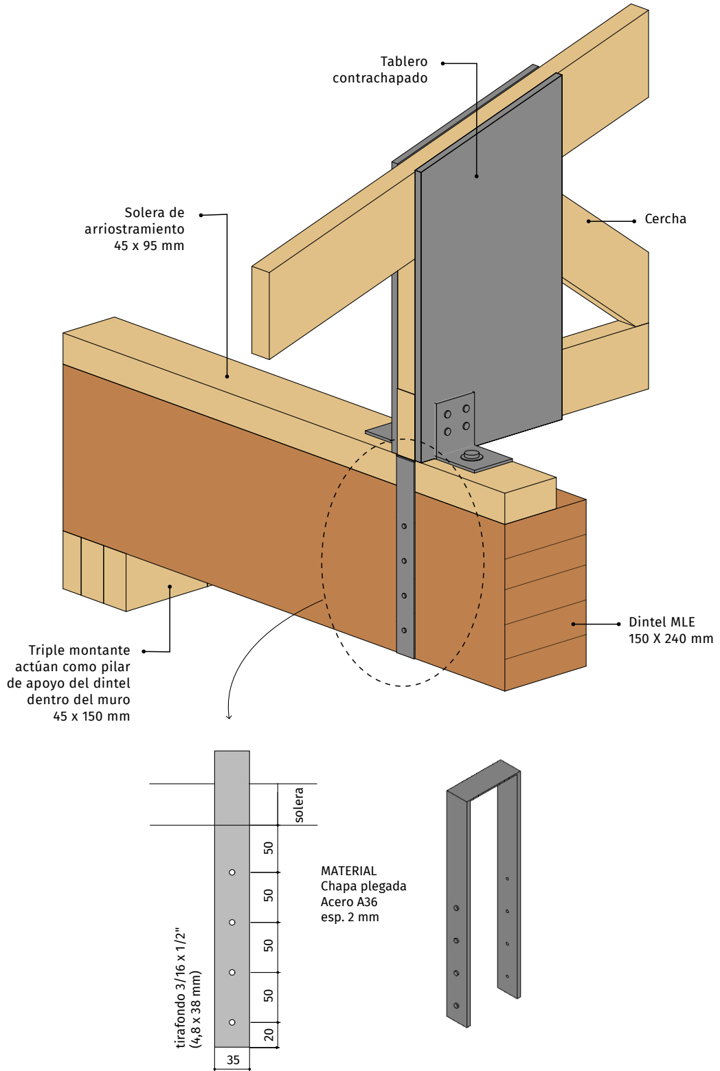
FIGURA 3.19. Detalle de apoyo de cercha sobre dintel de madera laminada
