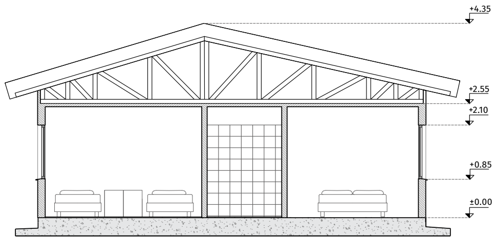
CORTE B-B
