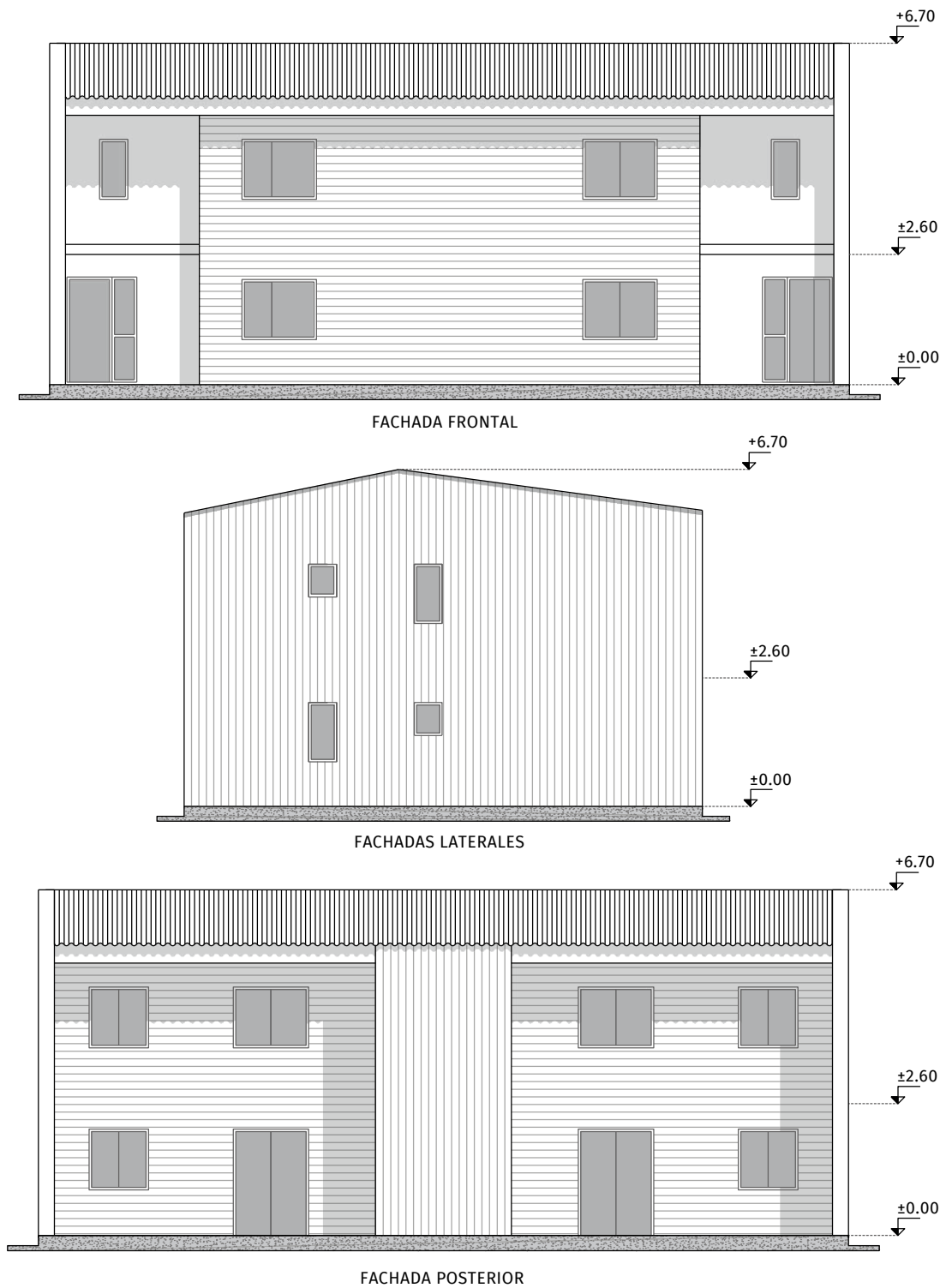
FIGURA 4.2 D Alzados
