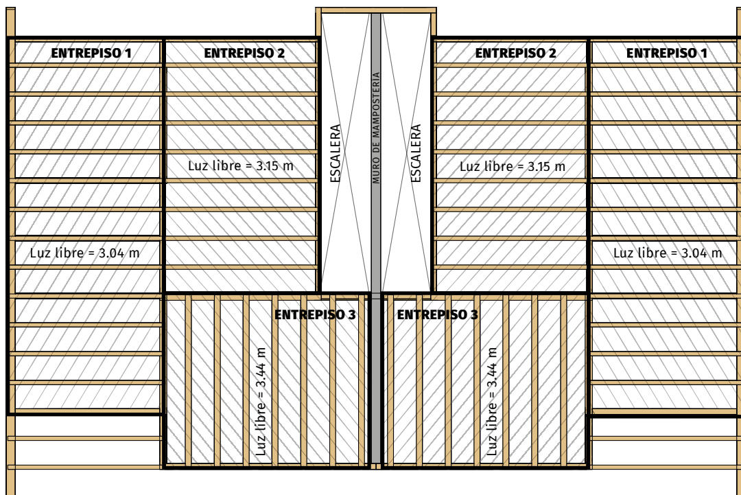
FIGURA 4.6 Esquema general de la estructura del entrepiso
