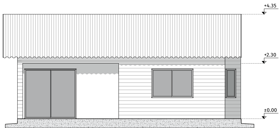
FACHADA POSTERIOR
