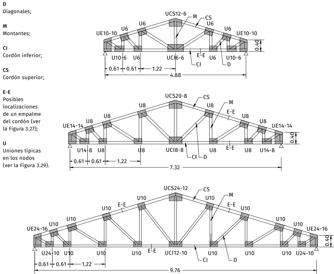
FIGURA 3.25 Descripción general de las cerchas con dos pendientes
