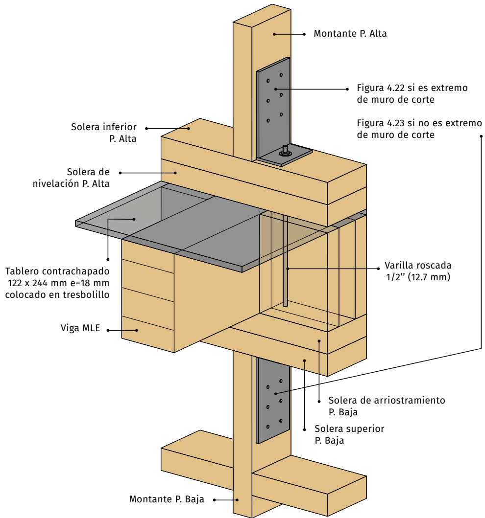
FIGURA 4.21 Detalle de conexión entre montantes de Planta Alta y Planta Baja para transmitir los esfuerzos de levantamiento originados por el viento
