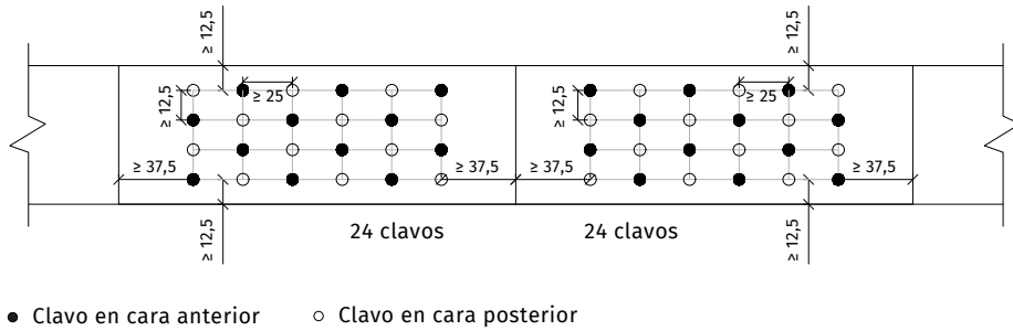
FIGURA 3.27. Detalles del empalme del cordón
