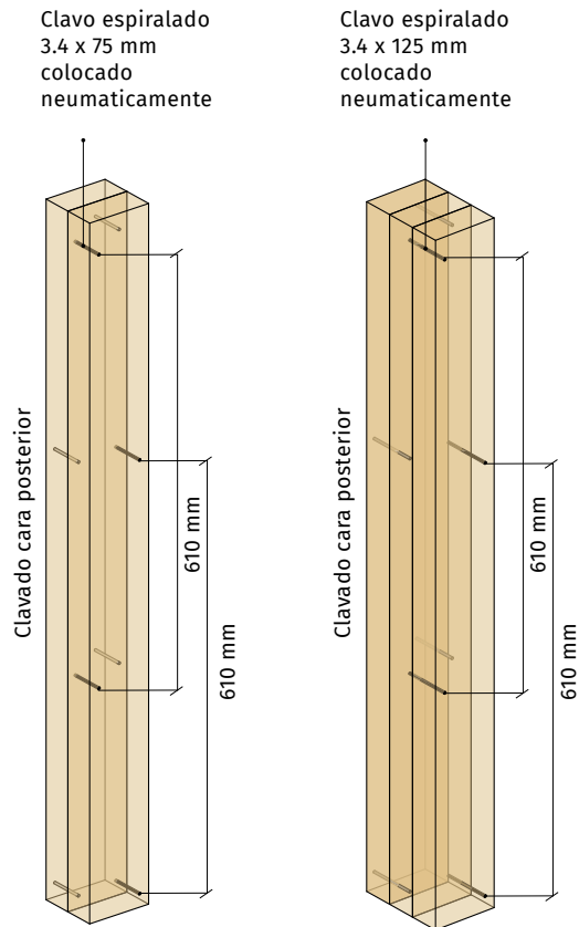
FIGURA 4.33 Unión de montantes constituidos por más de una pieza
