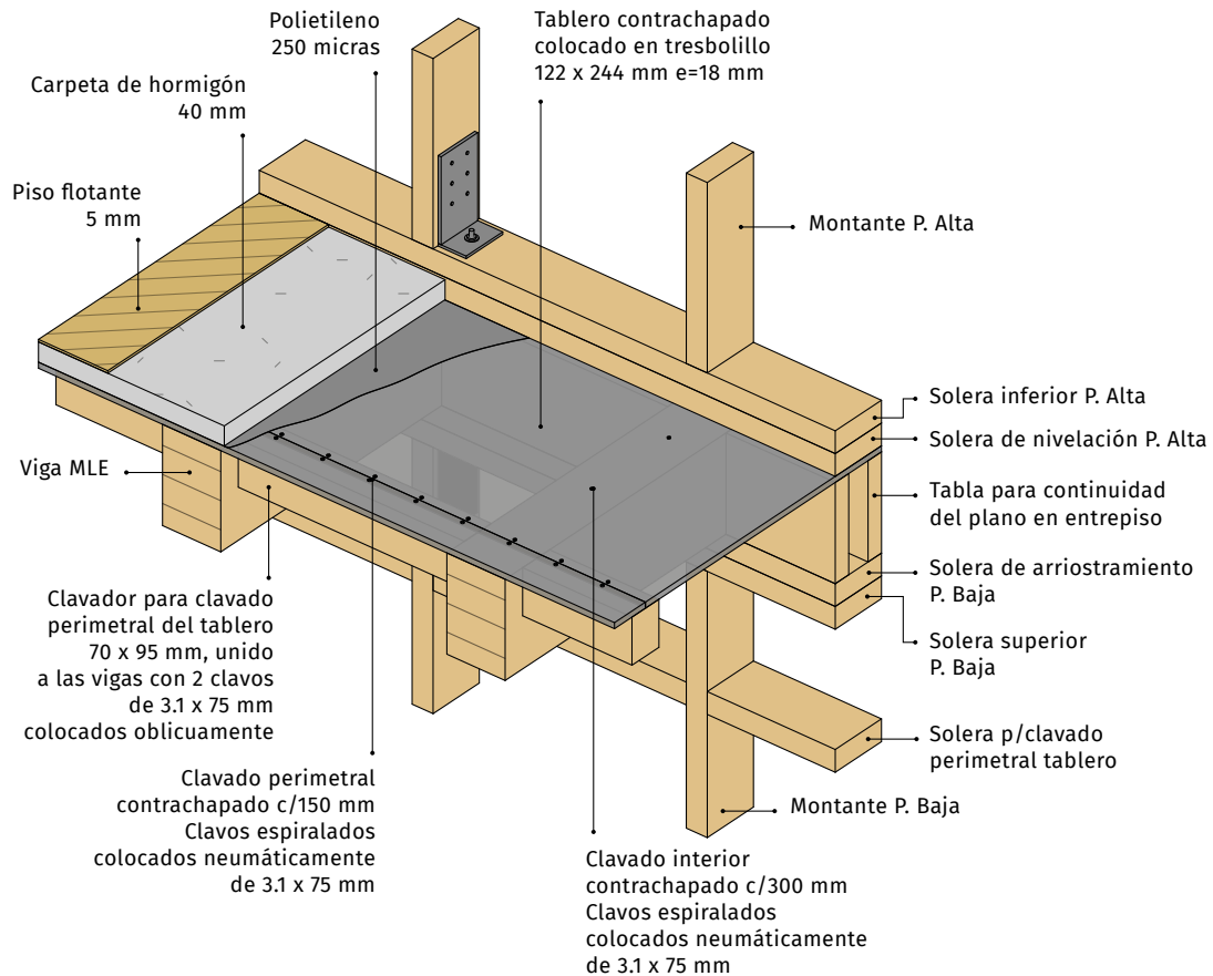
FIGURA 4.14 Detalle de la conformación del diafragma de entrepiso
