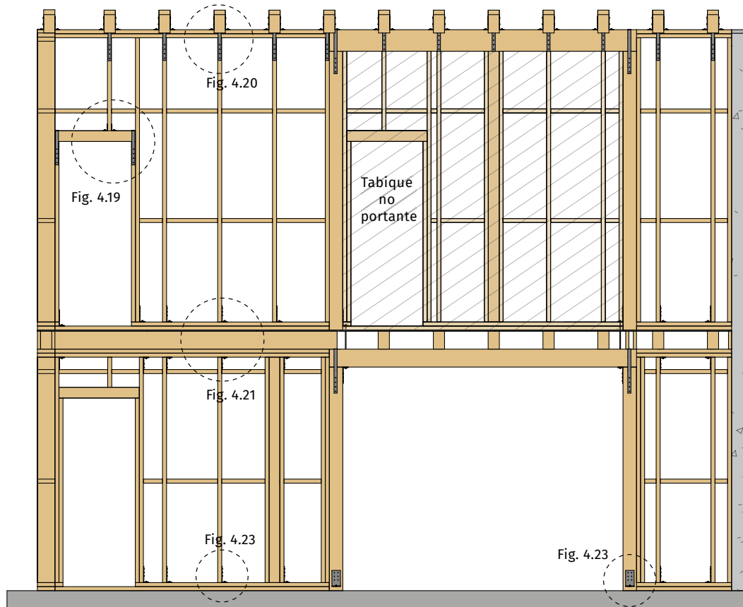
FIGURA 4.16 Conformación del muro interior de apoyo de la cubierta
