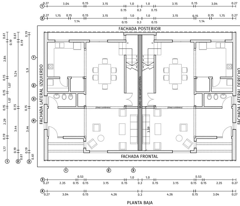
FIGURA 4.2 B Planta Baja
