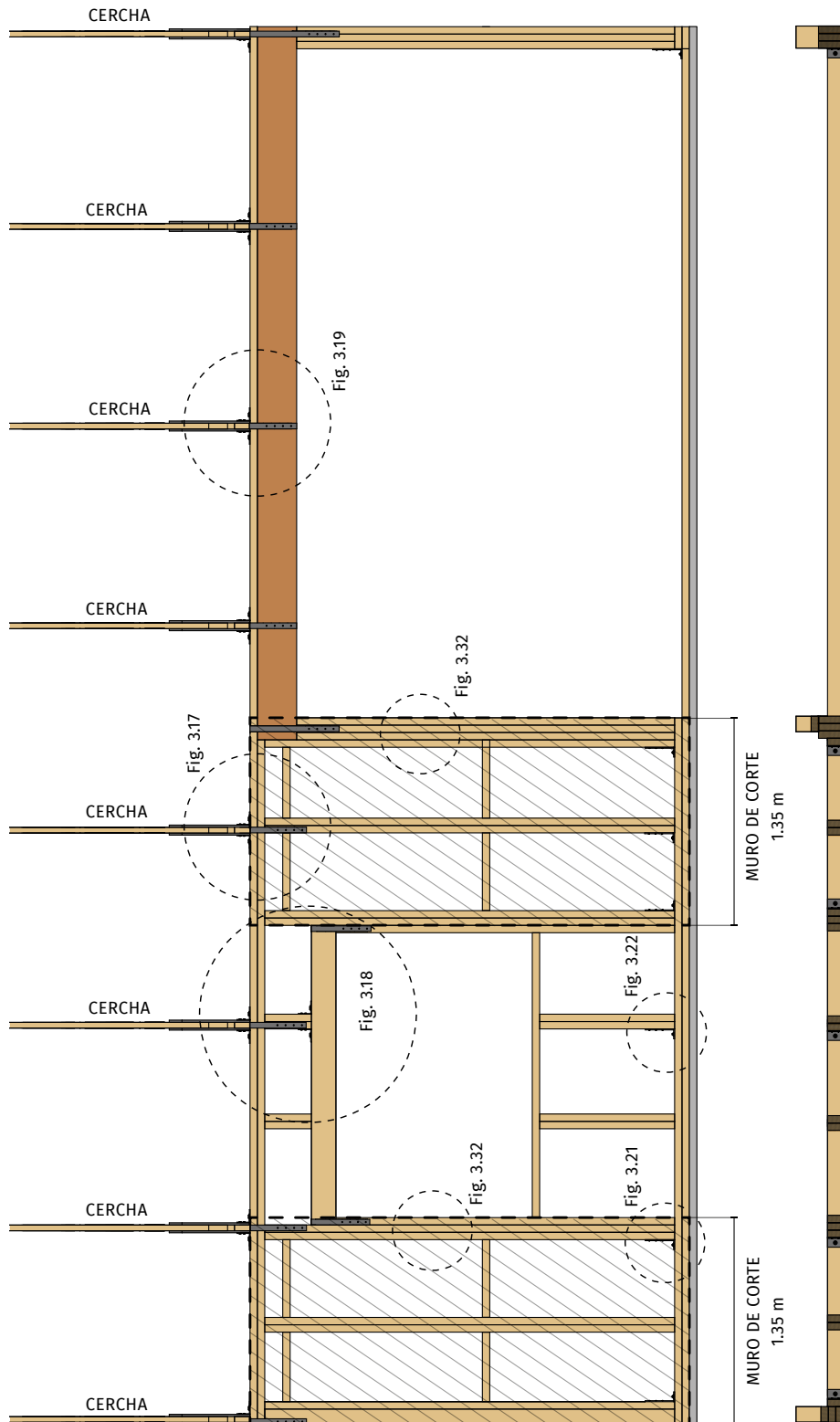
FIGURA 3.14. Conformación del muro de la fachada frontal
