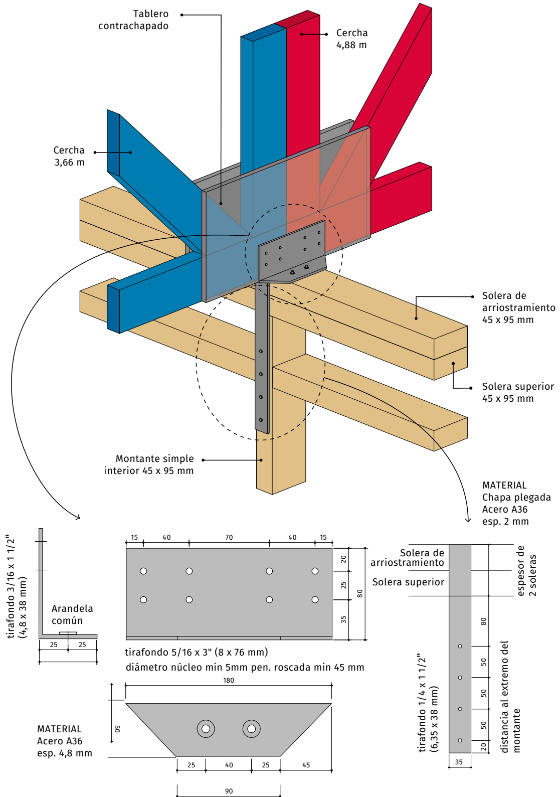
FIGURA 3.20. Detalle de unión de 2 cerchas concurrentes sobre el muro portante interior
