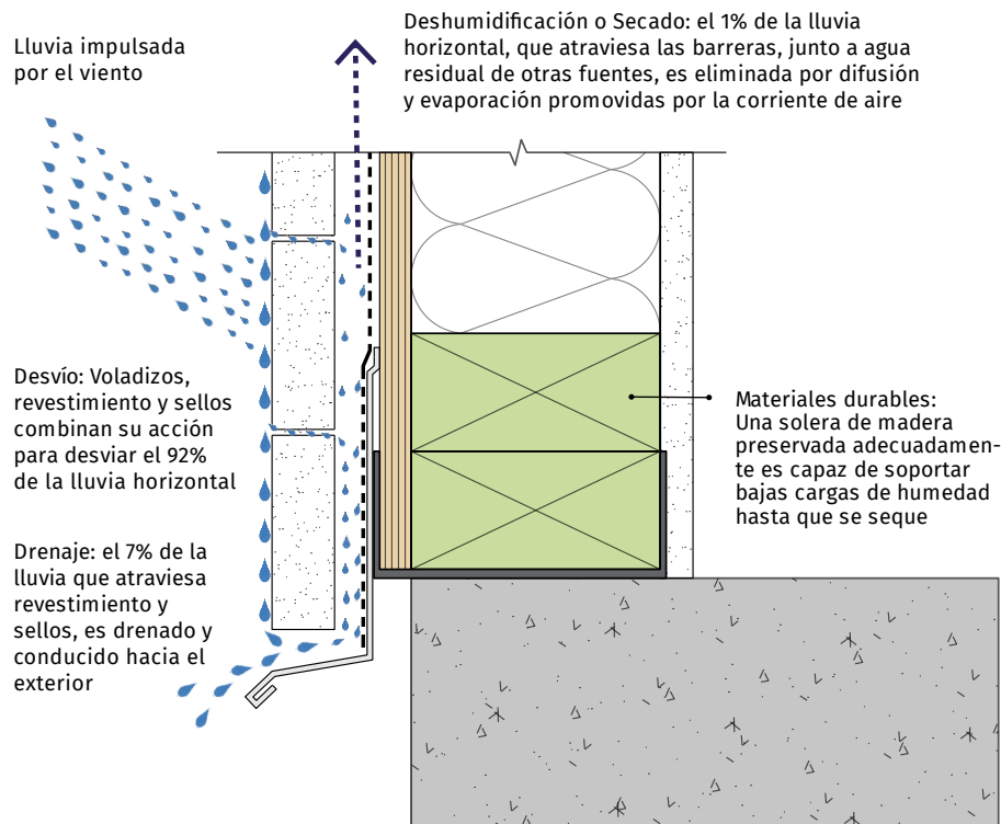
FIGURA 2.2. Ejemplo de aplicación de las estrategias de DESVÍO, DRENAJE, DESHUMIDIFICACIÓN Y MATERIALES DURABLES (adaptado de Think Wood, 2023)
