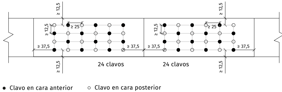
FIGURA 4.28 Detalles del empalme del cordón
