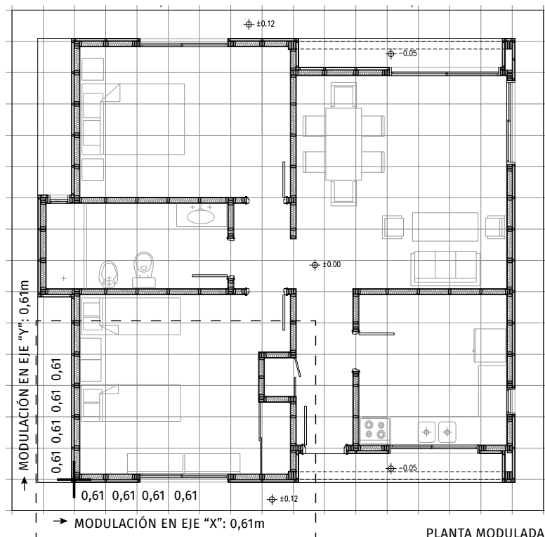
FIGURA 3.3. A. Modulación de entramado estructural
