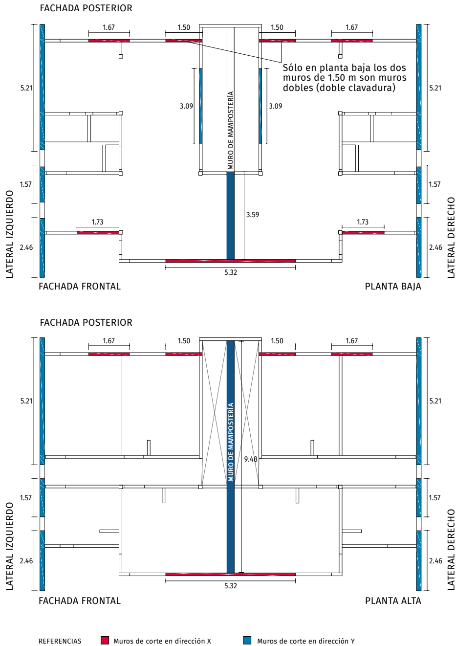
FIGURA 4.10 Longitud de muros de corte
