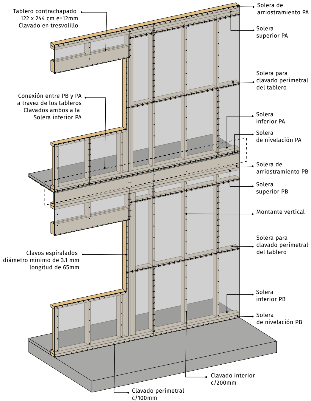
FIGURA 4.34 Clavado de los tableros a las soleras y montantes
