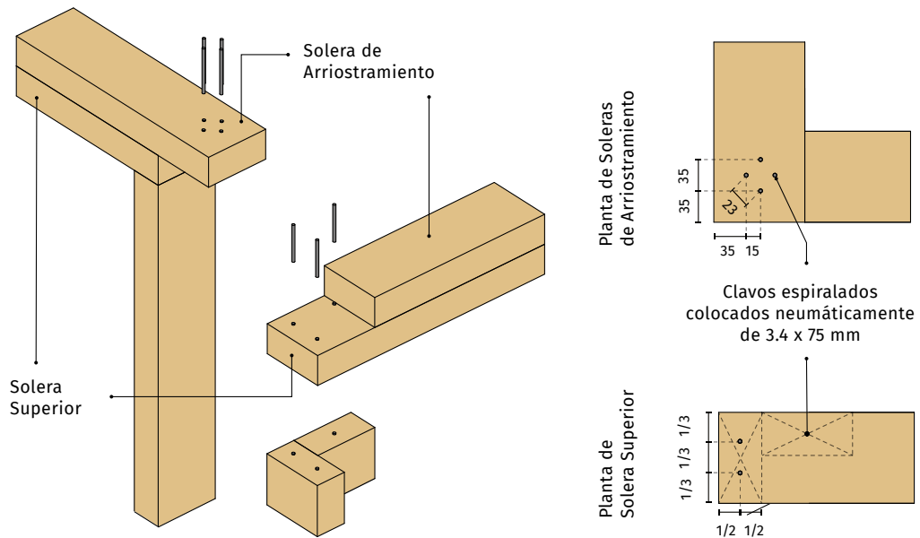
FIGURA 4.35 C. Clavadura de solera a montantes y entre soleras en esquina
