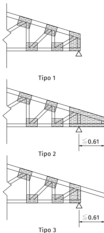
FIGURA 3.26. Tipologías de extremos
