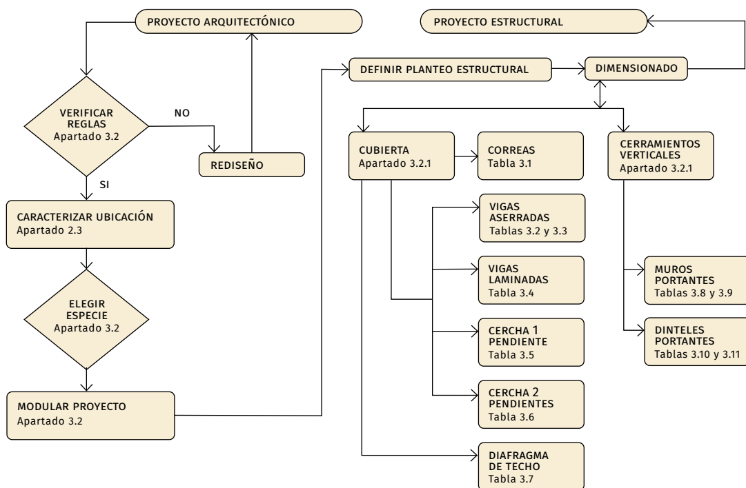
FIGURA 3.23. Diagrama de flujo del procedimiento general para resolución de la estructura
