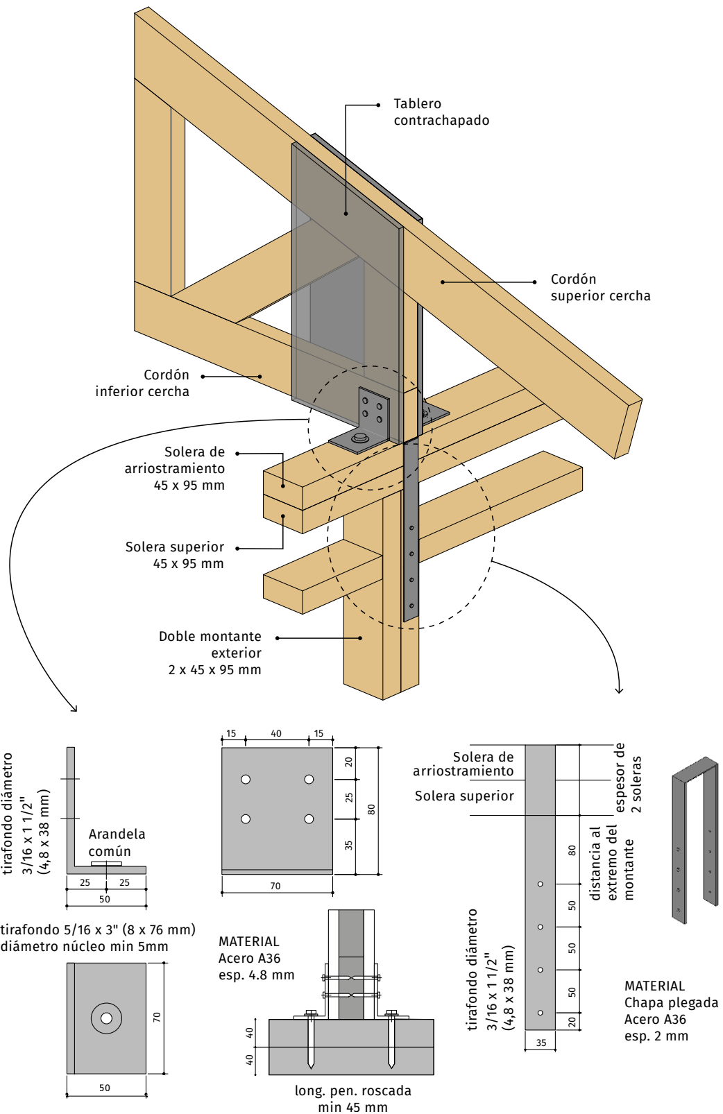
FIGURA 3.17. Detalle de la unión cercha-solera y solera-montante sobre los muros de ambas fachadas
