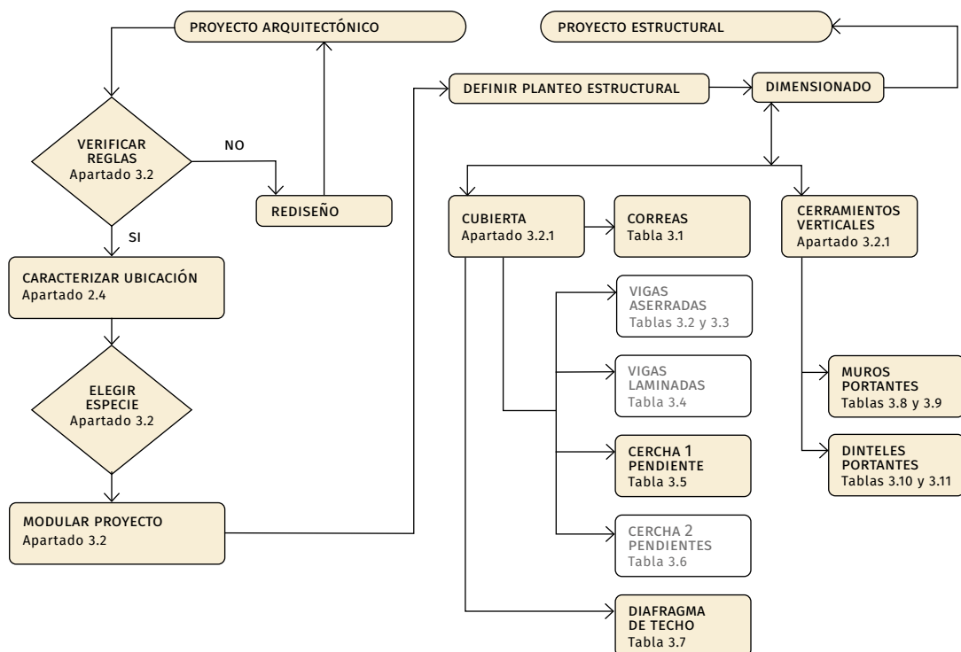
FIGURA 3.1. Diagrama de flujo del procedimiento adoptado para resolución del modelo
