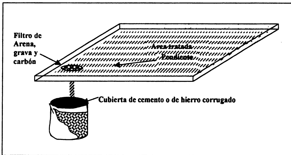
Figura 22. Sistemas de captación en áreas tratadas con pavimento u otros materiales.
