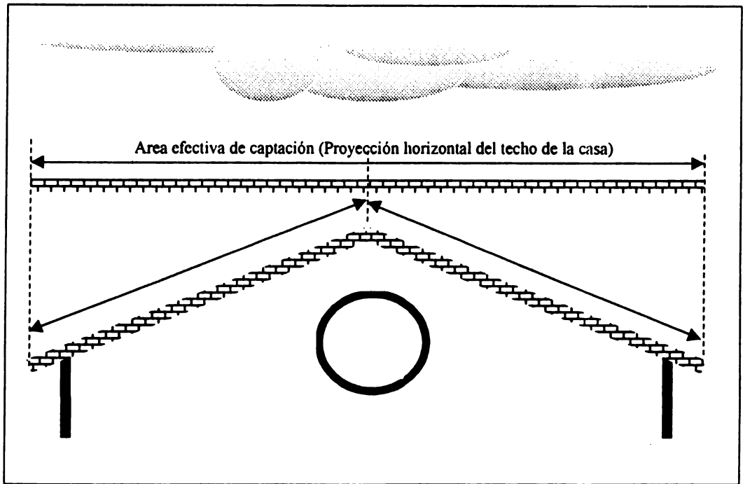
Figura 4. Área efectiva de captación.
