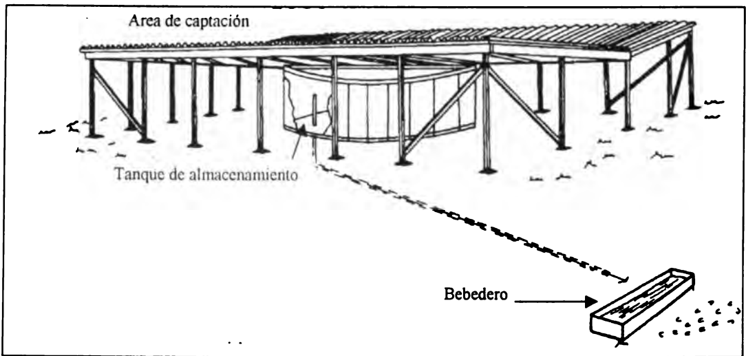
Figura 12. Techos cuenca para abrevaderos. (Velasco, 1977).
